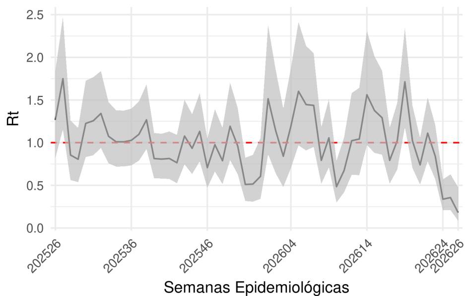
Figure 8: Número reprodutivo semanal de Dengue (a) e Chikungunya (b) para o município estimado até SE26.
