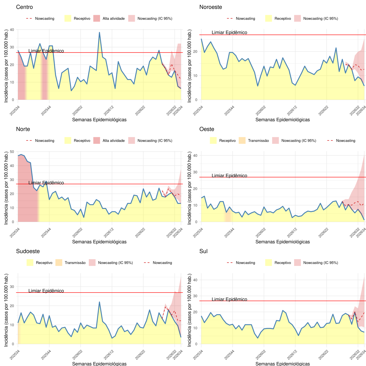
Figure 9: Curva de incidência de Dengue para os RPAs Centro, Norte e Sul até SE34. A linha azul representa o número de casos notificados e a linha vermelha horizontal o limiar epidêmico (incidência superior a 27 casos por 100 mil habitantes).
