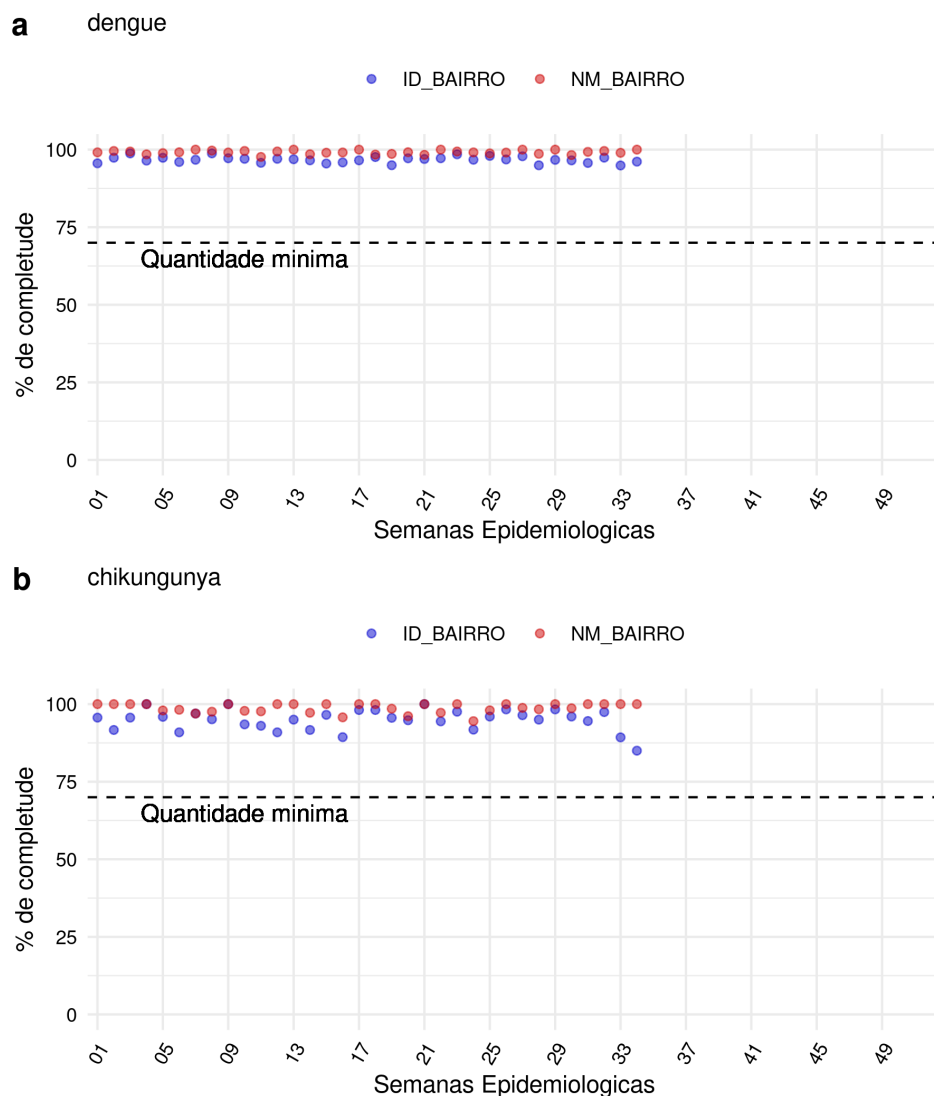
Figure 3: Completude dos dados notificados de Dengue (A) e Chikungunya (B) até a SE34 de acordo com as variáveis de identificação de bairro, nominal (NM_BAIRRO) e numérica (ID_BAIRRO).
