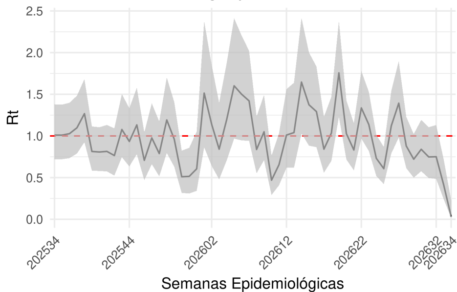
Figure 8: Número reprodutivo semanal de Dengue (a) e Chikungunya (b) para o município estimado até SE34.
