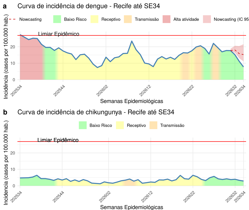
Figure 5: Curva de incidência de Dengue (A) e Chikungunya (B) - Recife/PE até SE34. A linha azul representa o número de casos observados e a linha vermelha horizontal o limiar epidêmico (incidência superior a 27 casos por 100 mil habitantes).
