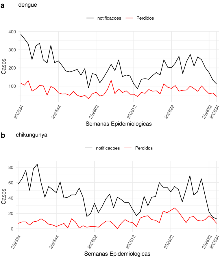
Figure 4: Número de dados notificados e perdidos de dengue (A) e chikungunya (B) até a SE34.
