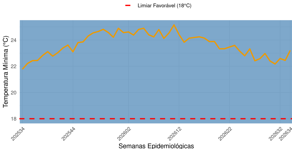
Figure 6: Receptividade climática e temperatura mínima do município até SE34. A linha amarela corresponde à variação da temperatura mínima durante o período. A área azul corresponde a período com receptividade climática favorável à transmissão de arboviroses, enquanto a área cinza a receptividade abaixo do limiar favorável.
