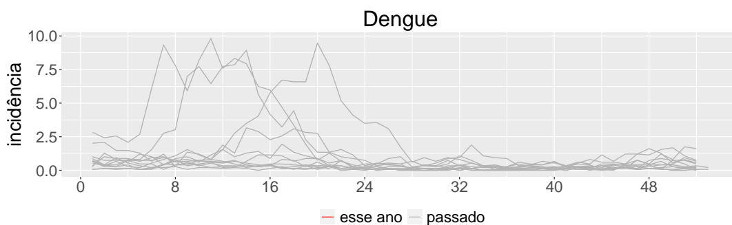
Figura 3. (A) Faixa azul claro indica o período com maior histórico de condições climáticas favoráveis para transmissão; (B) Média histórica do número reprodutivo na semana. Ocorrências isoladas de R > 1 não refletem transmissão sustentada; (C) Padrão sazonal da notificação de dengue nos últimos 10 anos. Em vermelho, a série deste ano.
