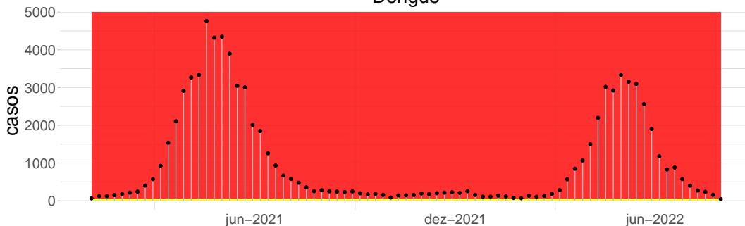
Dengue
