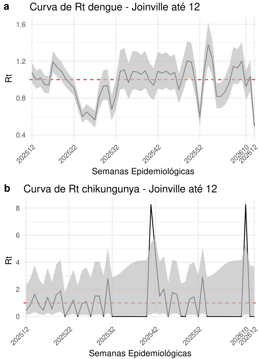
Figure 8: Número reprodutivo semanal de Dengue (a) e Chikungunya (b) para o município estimado até SE12.
