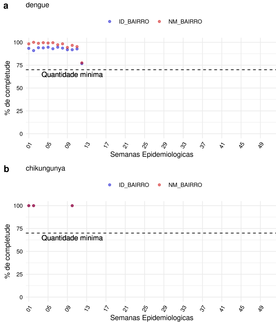
Figure 3: Completude dos dados notificados de Dengue (A) e Chikungunya (B) até a SE12de acordo com as variáveis de identificação de bairro, nominal (NM_BAIRRO) e numérica (ID_BAIRRO).
