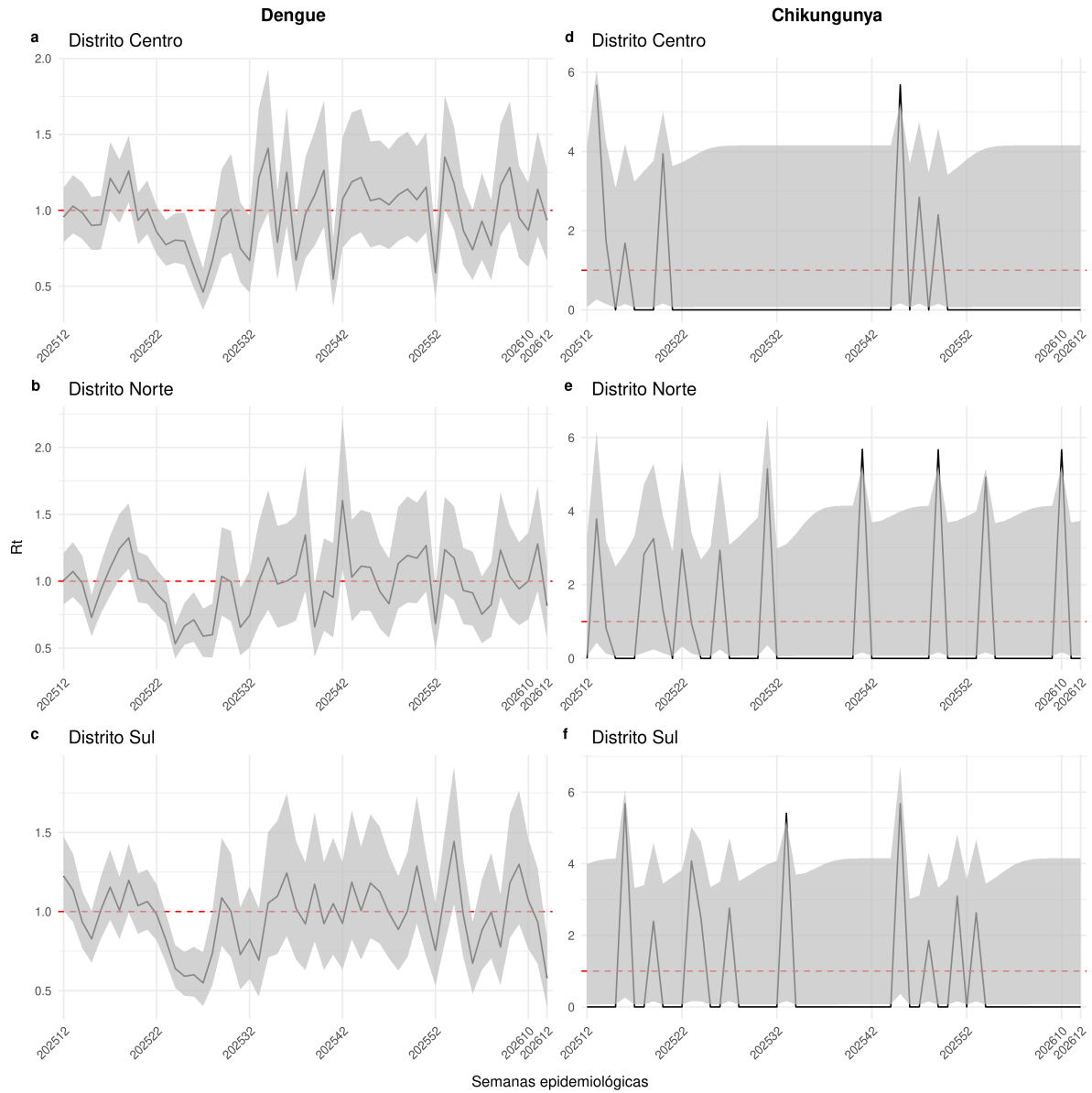
Figure 13: Número reprodutivo de dengue (a,b,c) e chikungunya (d,e,f) por RPA semanal estimado até SE12.
