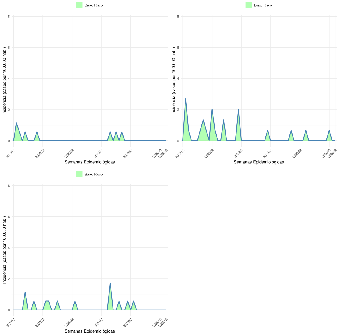
Figure 11: Curva de incidência de chikungunya para os RPAs Centro, Norte e Sul até SE12. A linha azul representa o número de casos notificados e a linha vermelha horizontal o limiar epidêmico (incidência superior a 27 casos por 100 mil habitantes).
