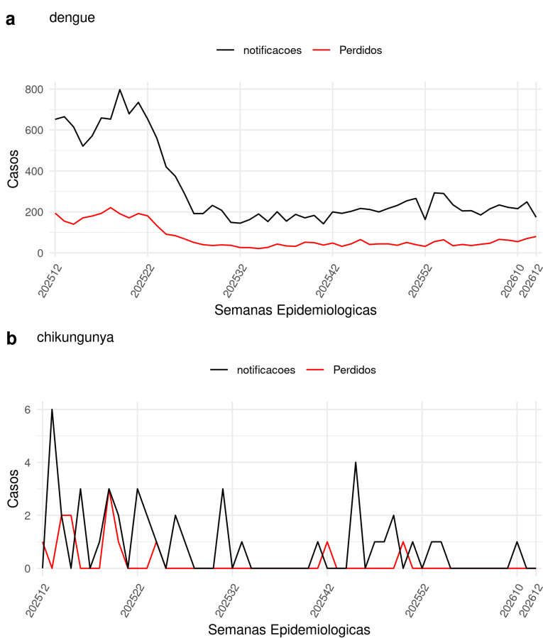
Figure 4: Número de dados notificados e perdidos de dengue (A) e chikungunya (B) até a SE12.
