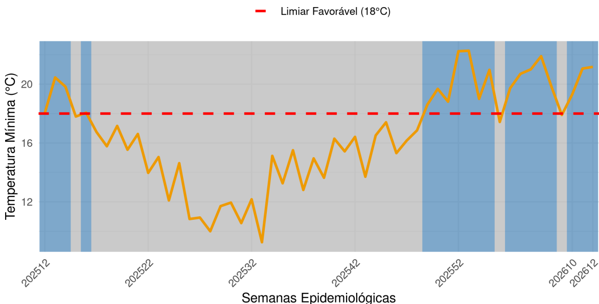
Figure 6: Receptividade climática e temperatura mínima do município até SE12. A linha amarela corresponde à variação da temperatura mínima durante o período. A área azul corresponde a período com receptividade climática favorável à transmissão de arboviroses, enquanto a área cinza a receptividade abaixo do limiar favorável.
