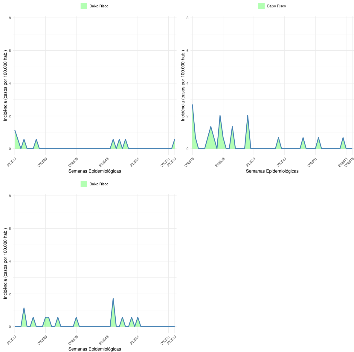
Figure 11: Curva de incidência de chikungunya para os RPAs Centro, Norte e Sul até SE13. A linha azul representa o número de casos notificados e a linha vermelha horizontal o limiar epidêmico (incidência superior a 27 casos por 100 mil habitantes).
