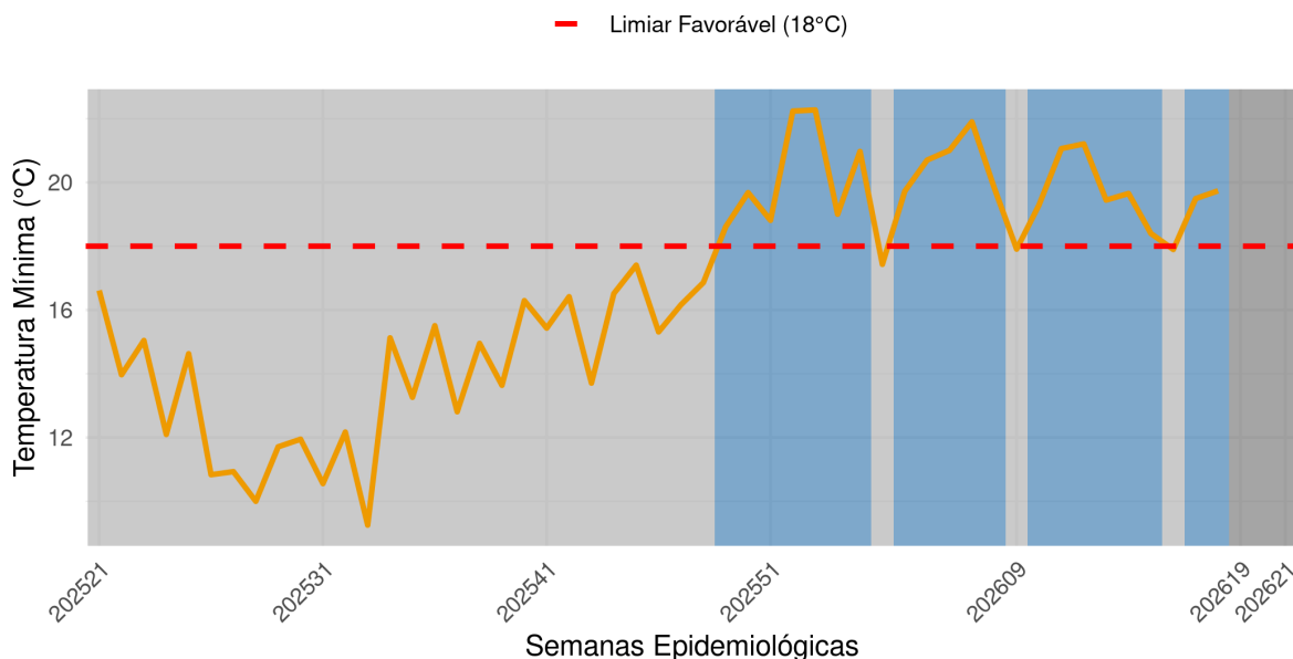
Figure 6: Receptividade climática e temperatura mínima do município até SE21. A linha amarela corresponde à variação da temperatura mínima durante o período. A área azul corresponde a período com receptividade climática favorável à transmissão de arboviroses, enquanto a área cinza a receptividade abaixo do limiar favorável.
