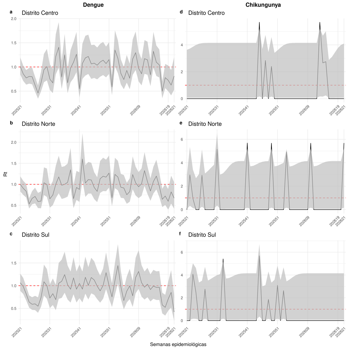
Figure 13: Número reprodutivo de dengue (a,b,c) e chikungunya (d,e,f) por RPA semanal estimado até SE21.
