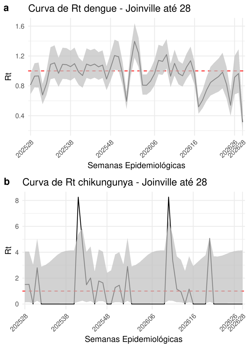
Figure 8: Número reprodutivo semanal de Dengue (a) e Chikungunya (b) para o município estimado até SE28.
