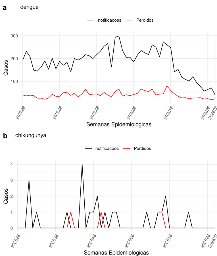
Figure 4: Número de dados notificados e perdidos de dengue (A) e chikungunya (B) até a SE28.
