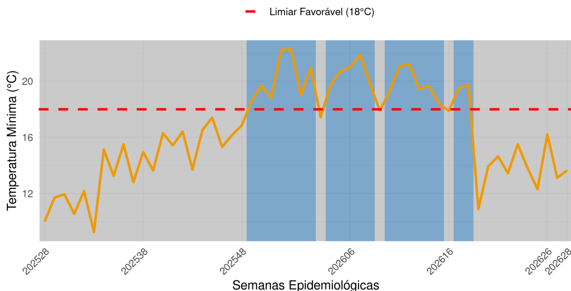
Figure 6: Receptividade climática e temperatura mínima do município até SE28. A linha amarela corresponde à variação da temperatura mínima durante o período. A área azul corresponde a período com receptividade climática favorável à transmissão de arboviroses, enquanto a área cinza a receptividade abaixo do limiar favorável.
