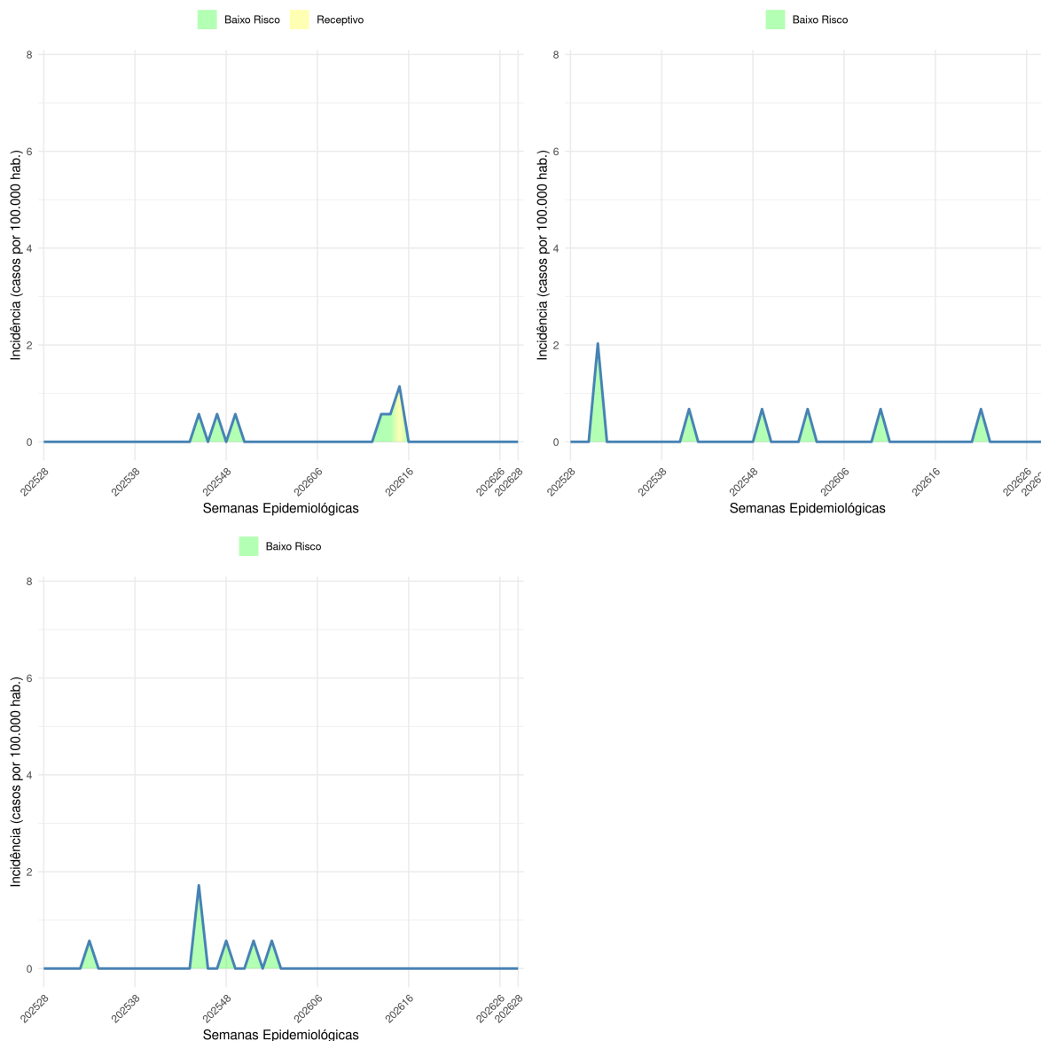
Figure 11: Curva de incidência de chikungunya para os RPAs Centro, Norte e Sul até SE28. A linha azul representa o número de casos notificados e a linha vermelha horizontal o limiar epidêmico (incidência superior a 27 casos por 100 mil habitantes).
