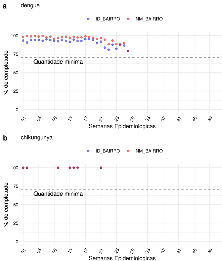
Figure 3: Completude dos dados notificados de Dengue (A) e Chikungunya (B) até a SE28de acordo com as variáveis de identificação de bairro, nominal (NM_BAIRRO) e numérica (ID_BAIRRO).
